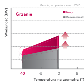
30% wzrost wydajności (Porównanie z konwencjonalnym)
