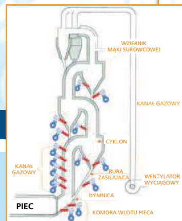
Wieża wymienników w cementowni
