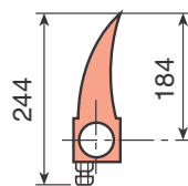
Ostrze czyszczące
